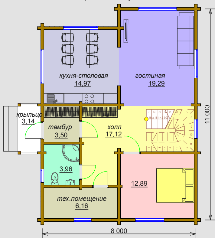
План 1го этажа S = 77,9 м2 без крыльца
