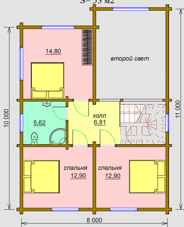
План 2го этажа S= 53 м2
